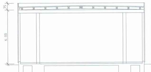
SCHNITT B-B
